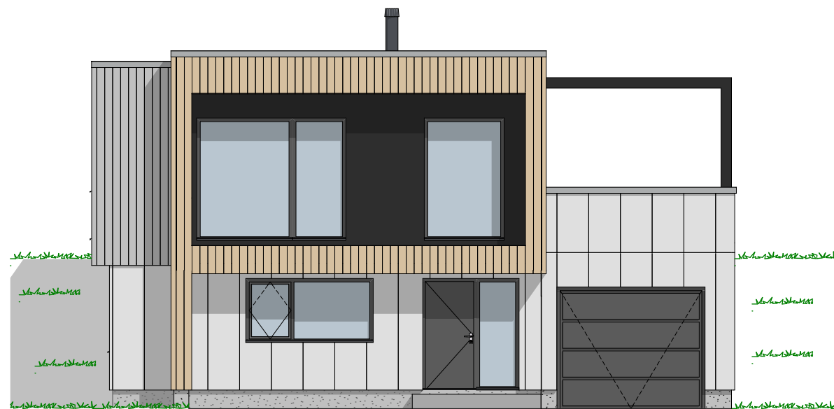
1:100 Fasade Sør Vest
