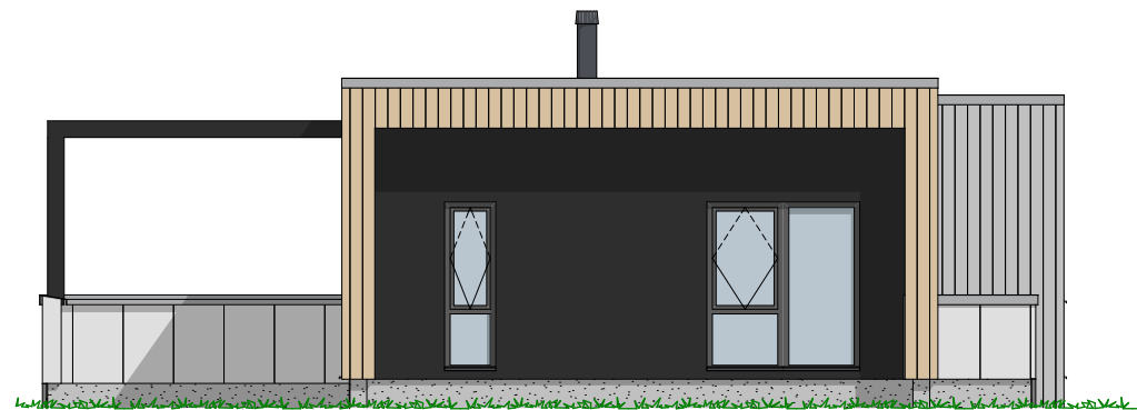
1:100 Fasade Nord Øst
