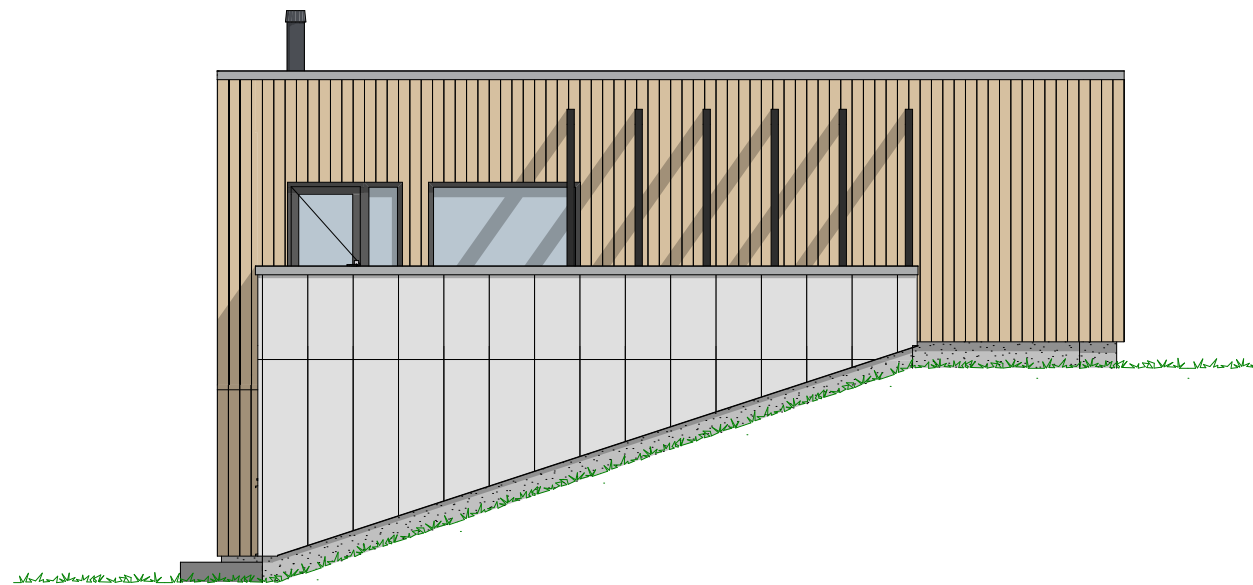
1:100 Fasade Sør Øst
