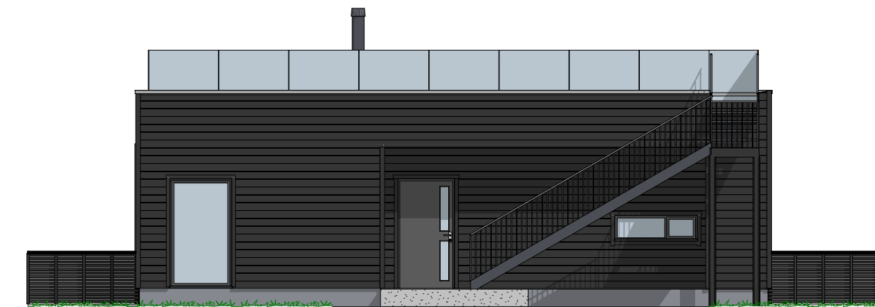
1:100 Fasade Nord
