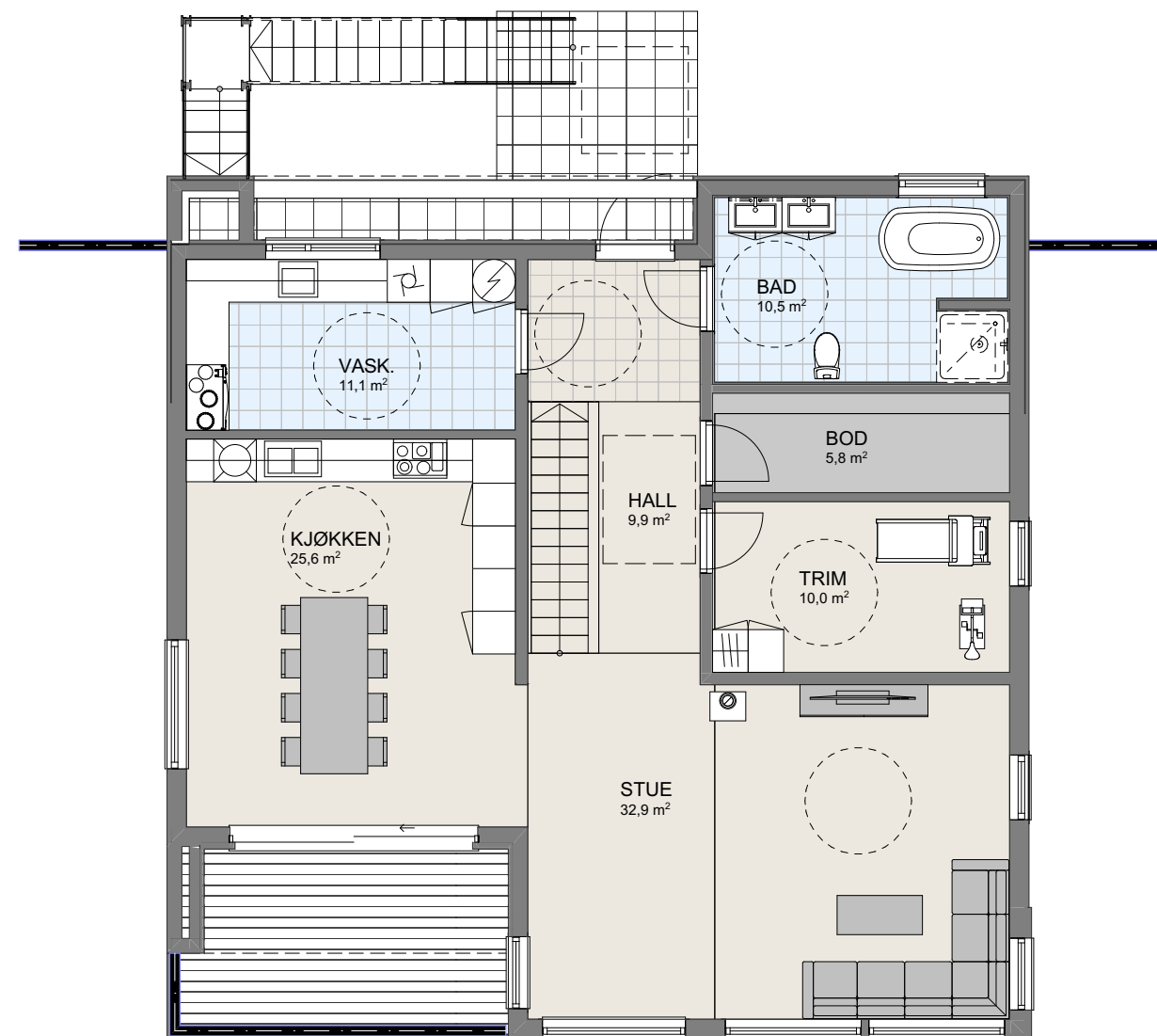
1:100 H.Etasje
