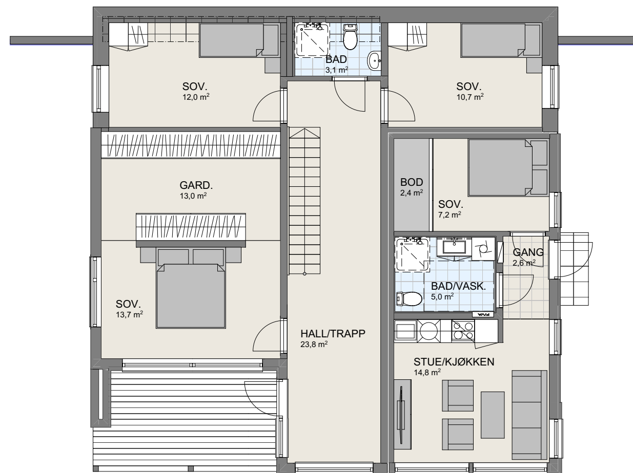
1:100 U. Etasje
