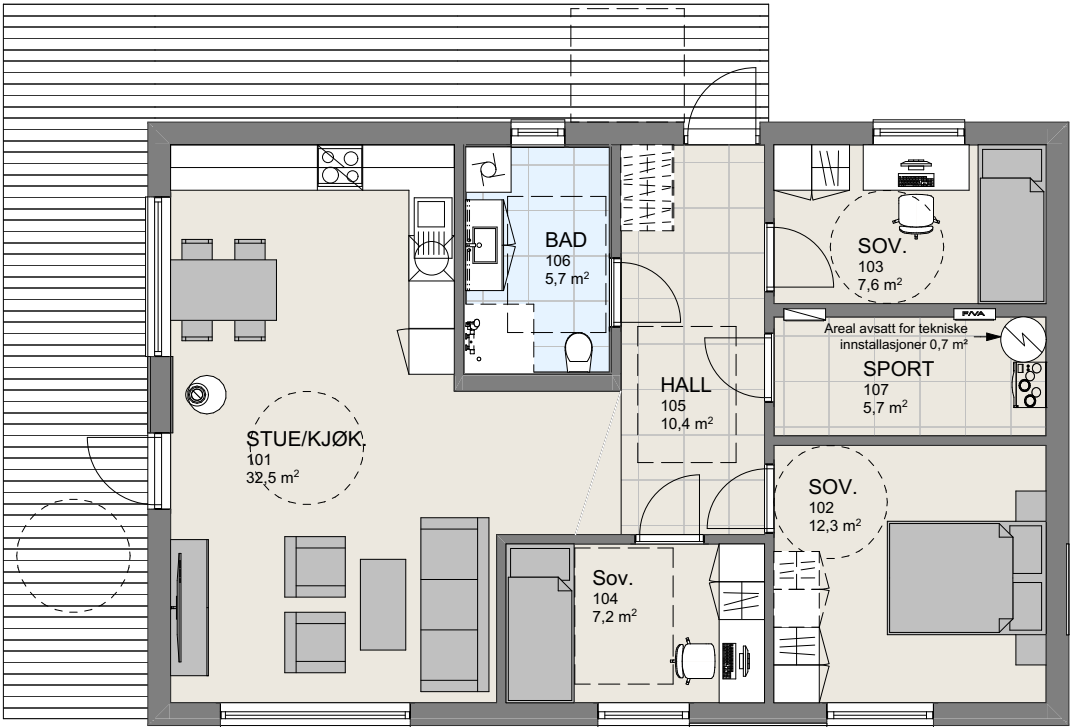
1:100 H. Etasje
