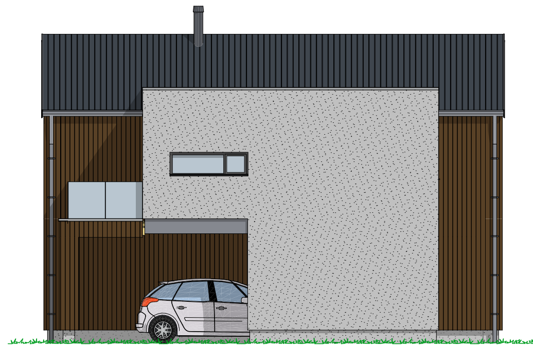
1:100 Fasade Øst
