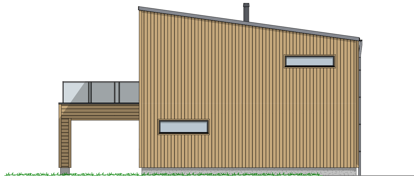
1:100 Fasade Nord-øst
