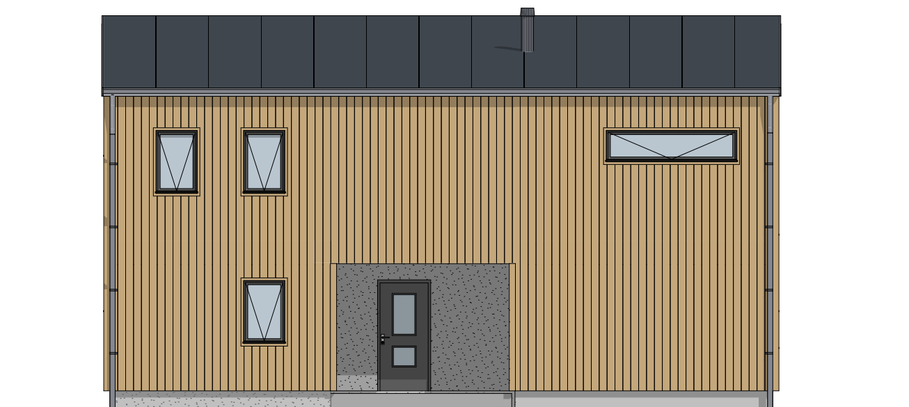
1:100 Fasade Nord-vest
