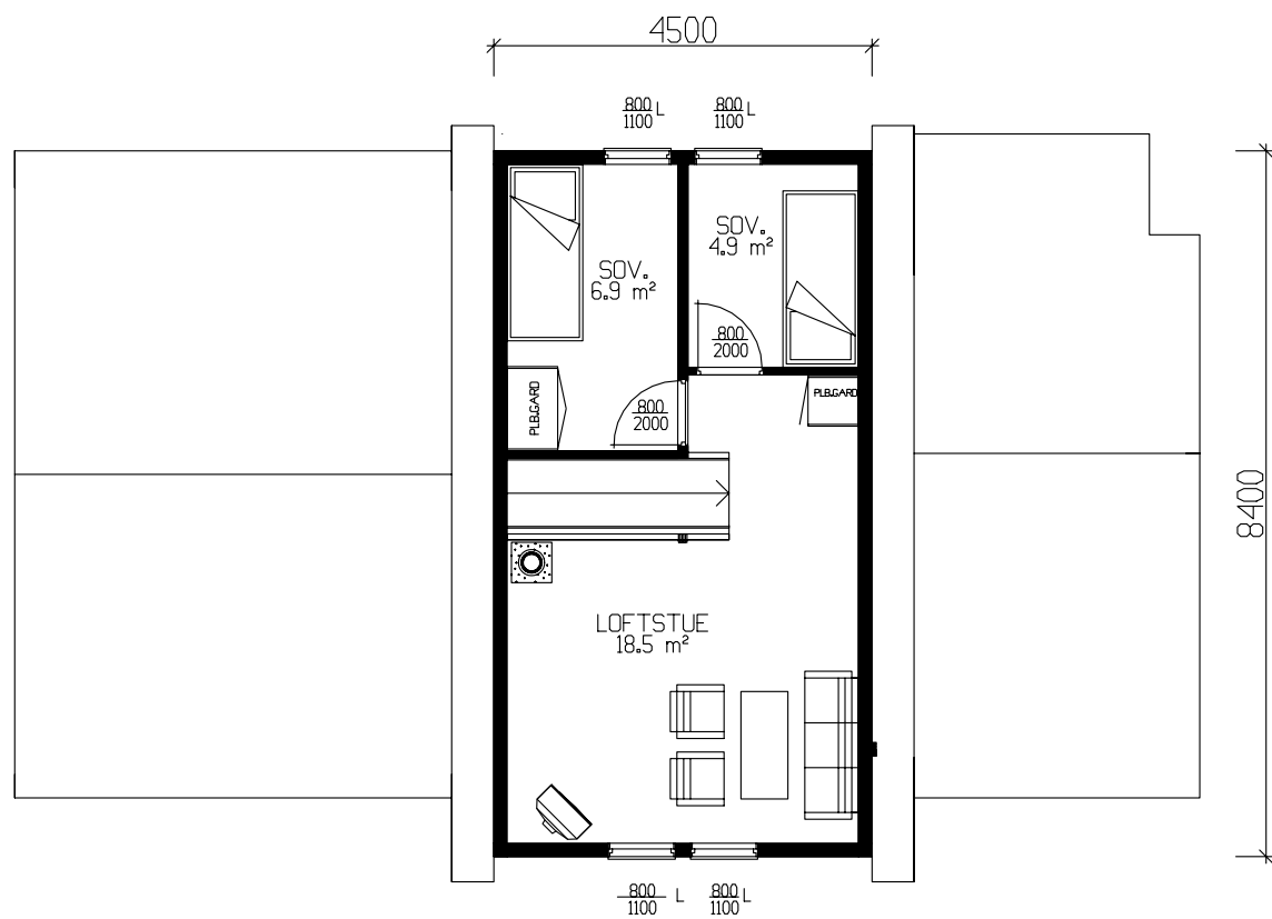
LOFTSPLAN 33,8m² BRA
