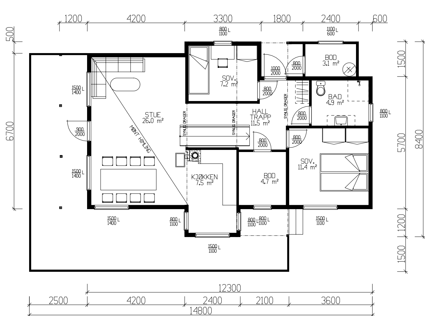
HOVEDPLAN 75,6m² BRA + BOD 3,1m²
