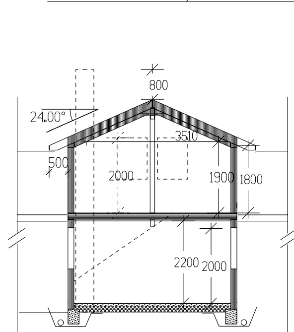
SNITT-LOFTSTUE
