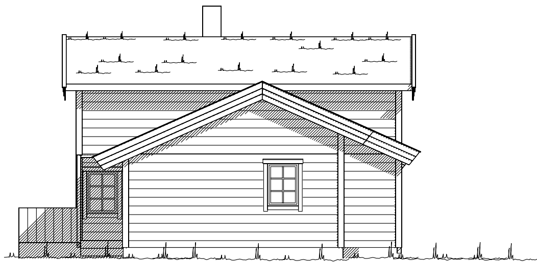
Fasade mot
