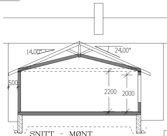
SNITT - MØNT
