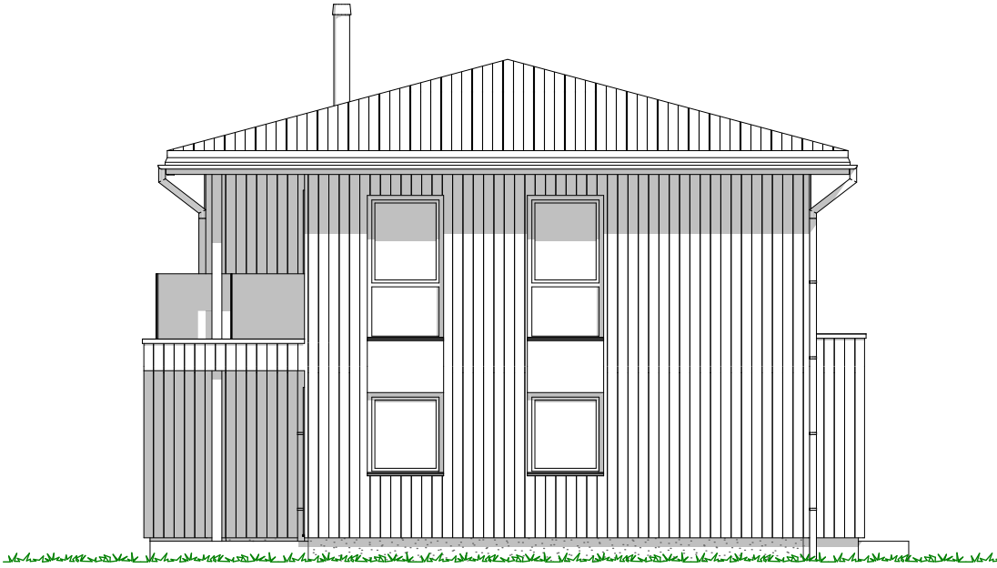
1:100 Fasade Nord Vest
