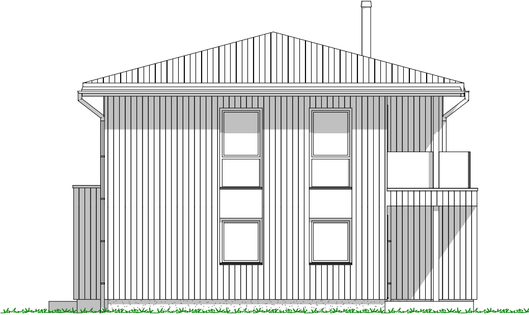
1:100 Fasade Sør Øst
