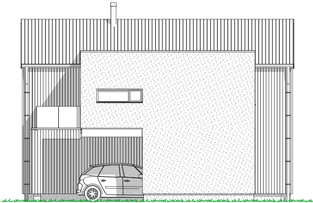
1:100 Fasade Øst
