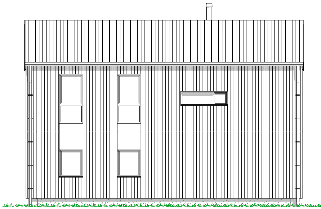
1:100 Fasade Vest
