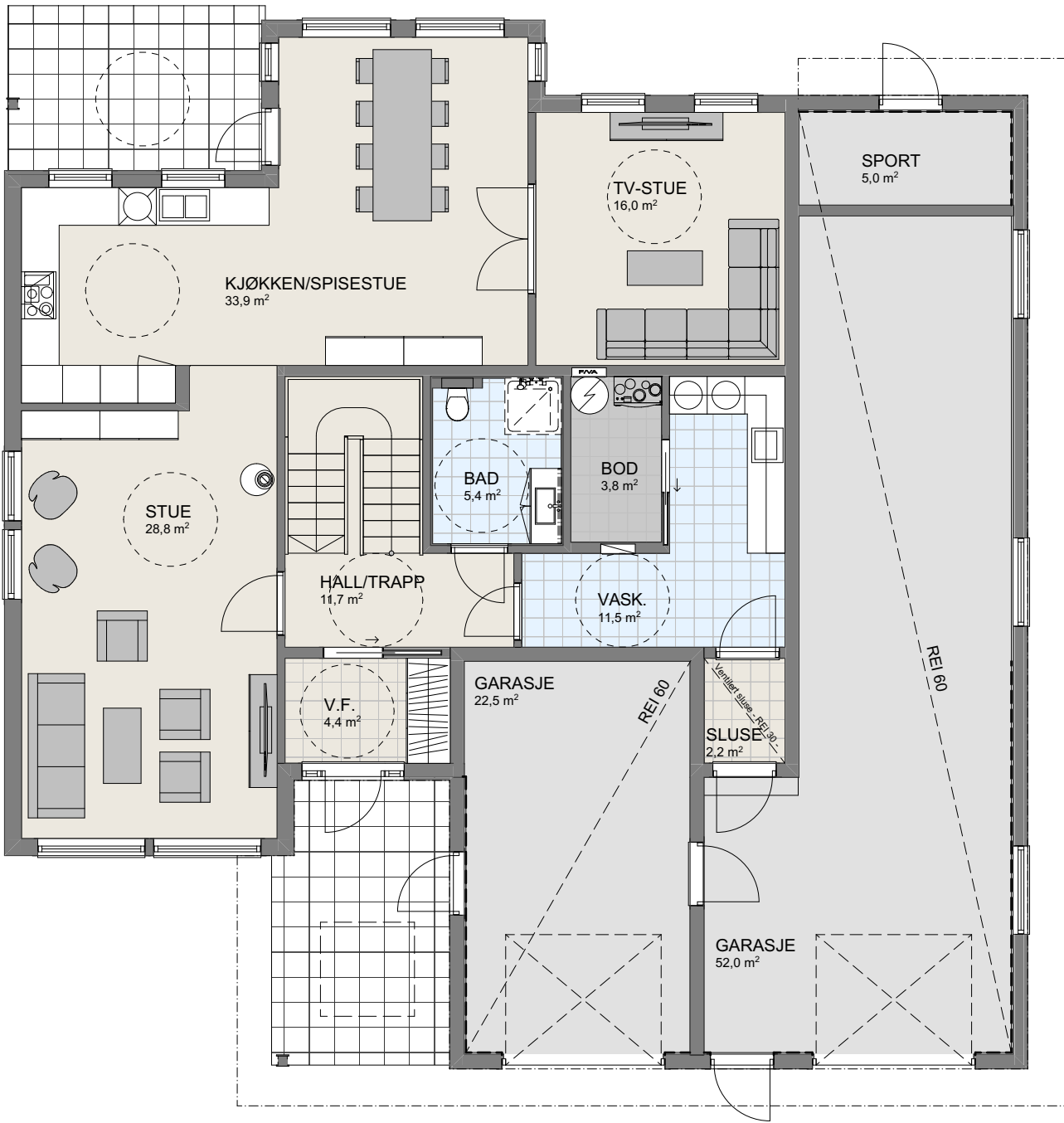
1:100 H. Etasje
