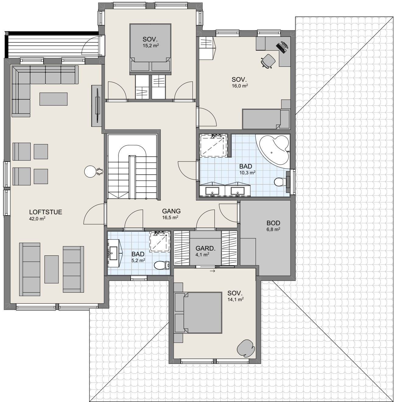
1:100 2.Etasje
