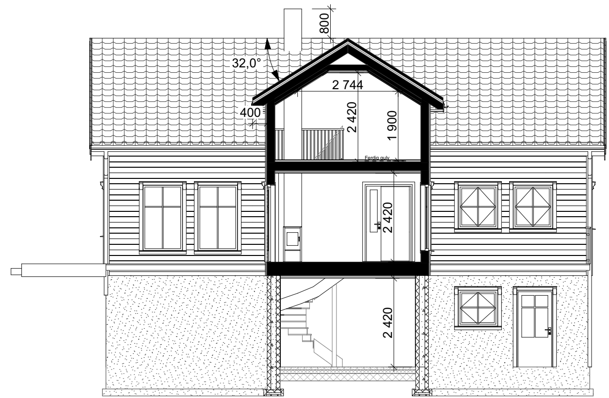
1:100 Snitt B
