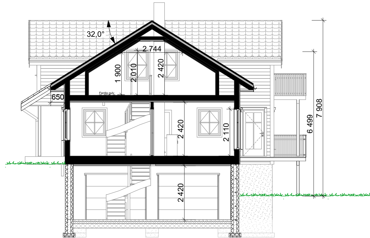
1:100 Snitt A
