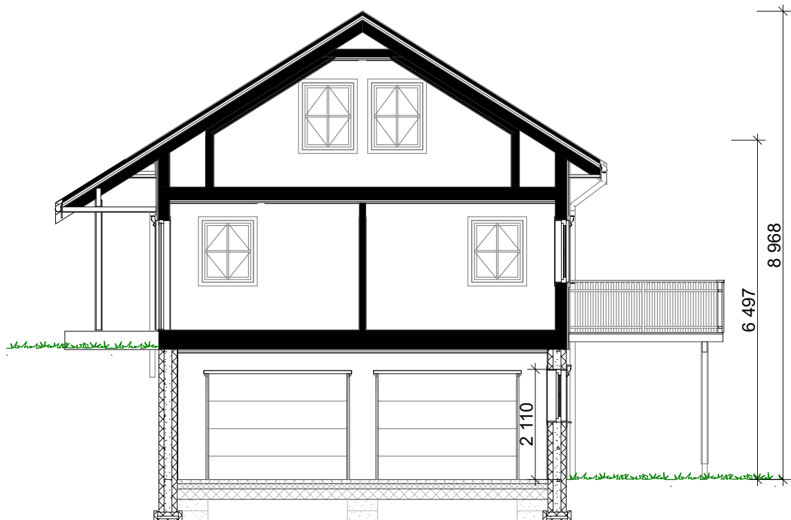
1:100 Snitt C
