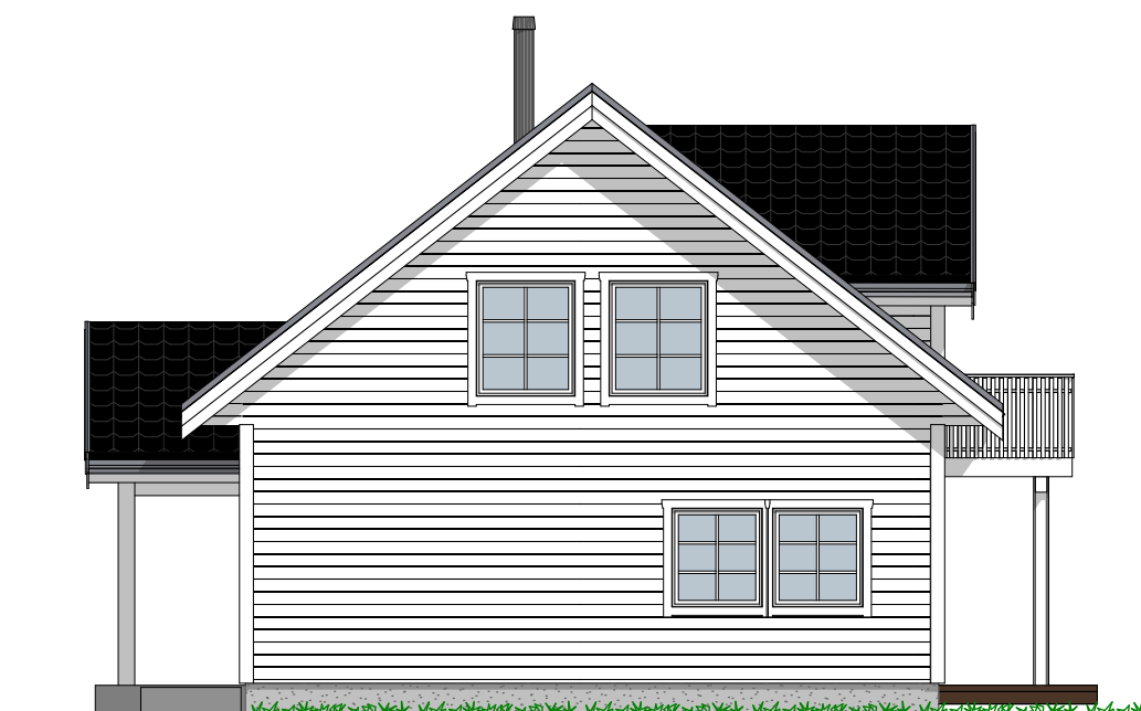
1:100 Fasade Nord
