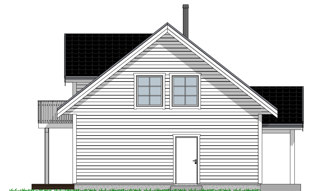
1:100 Fasade Sør
