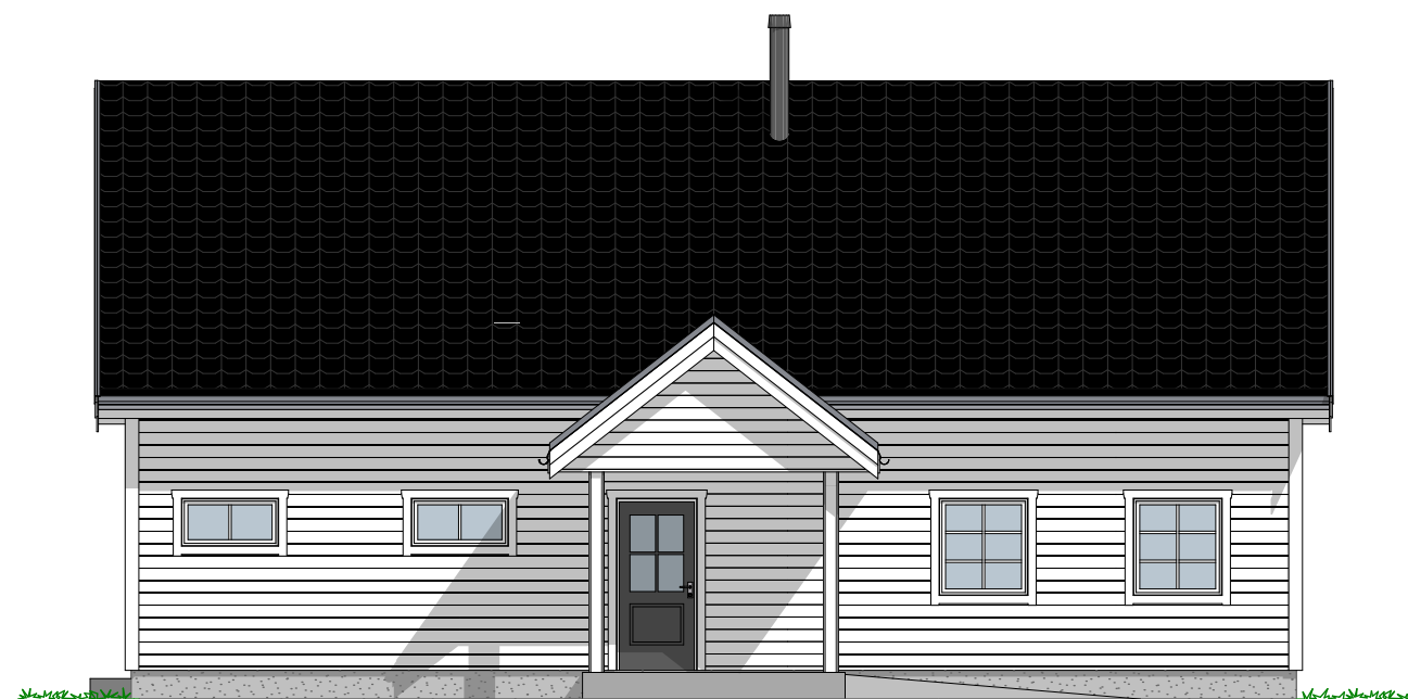
1:100 Fasade Øst
