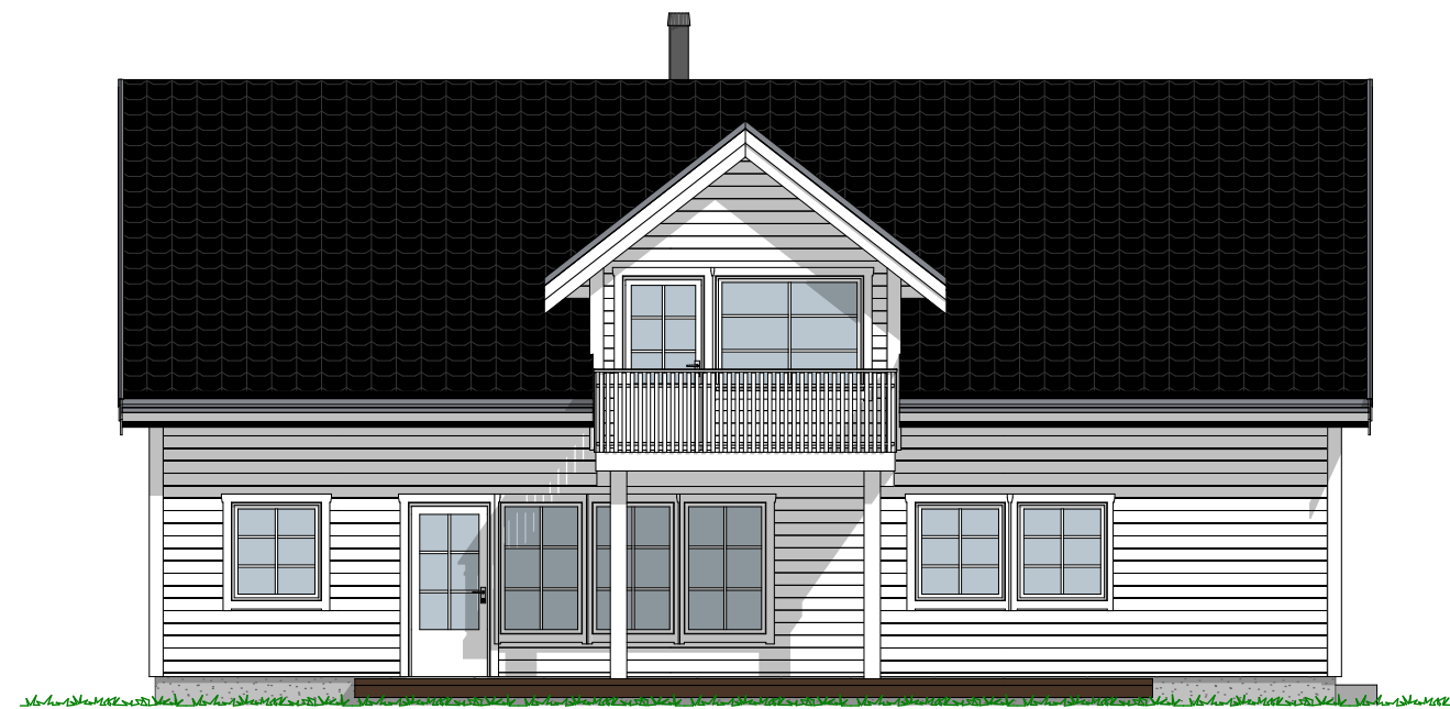
1:100 Fasade Vest
