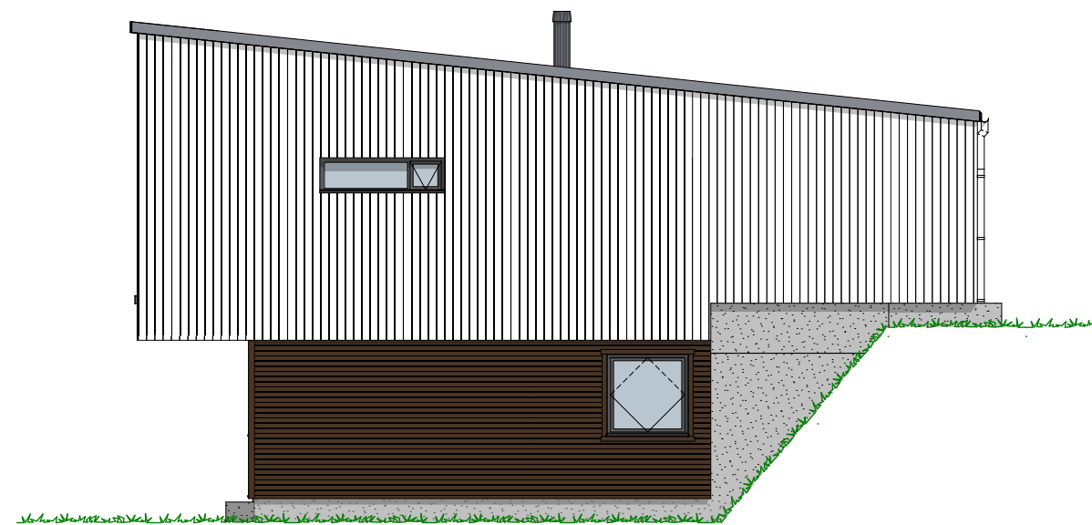
1:100 Fasade Øst
