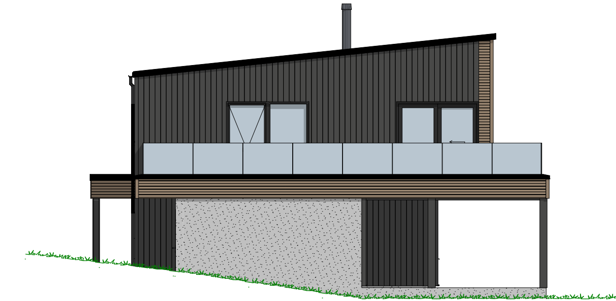
1:100 Fasade Nord
