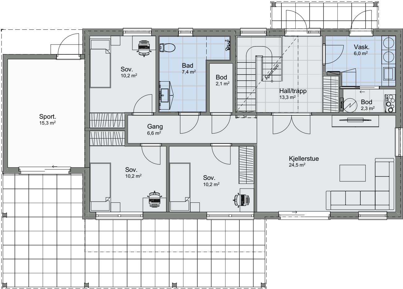
1:100 H. etasje
