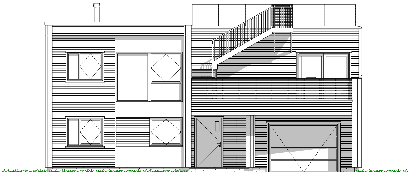
1:100 Fasade Sør Sør Vest
