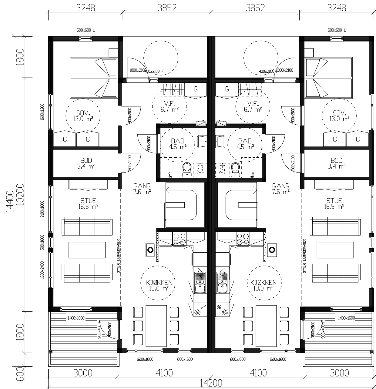
HOVEDPLAN 77,3m² BRA PR LEILIGHET
