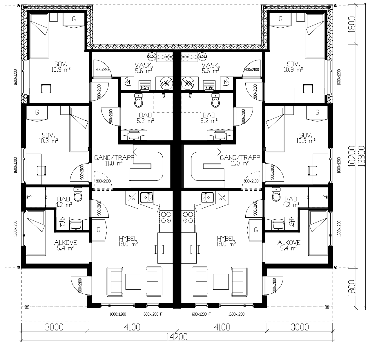
UNDERETASJE 75,4m² BRA PR LEILIGHET
