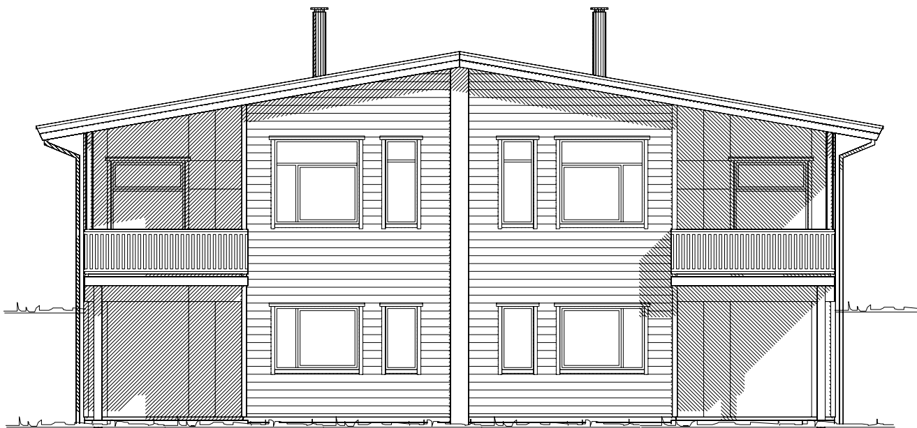
Fasade mot _____.
