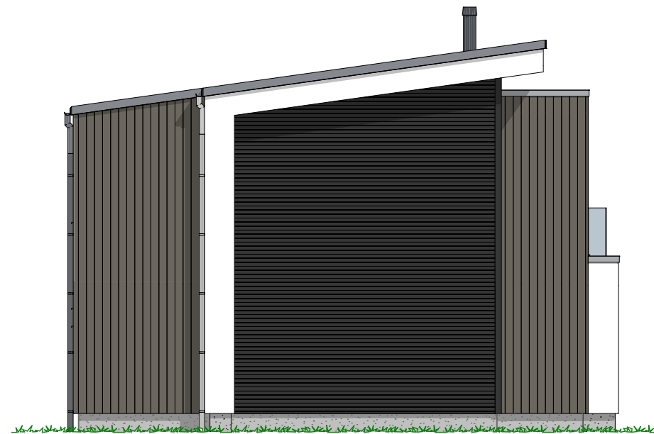
1:100 Fasade Nord Vest
