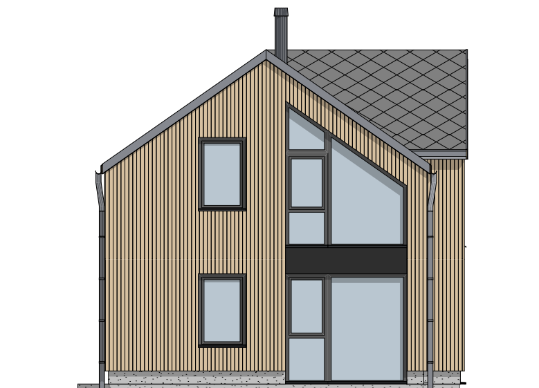
1:100 Fasade Sør Vest
