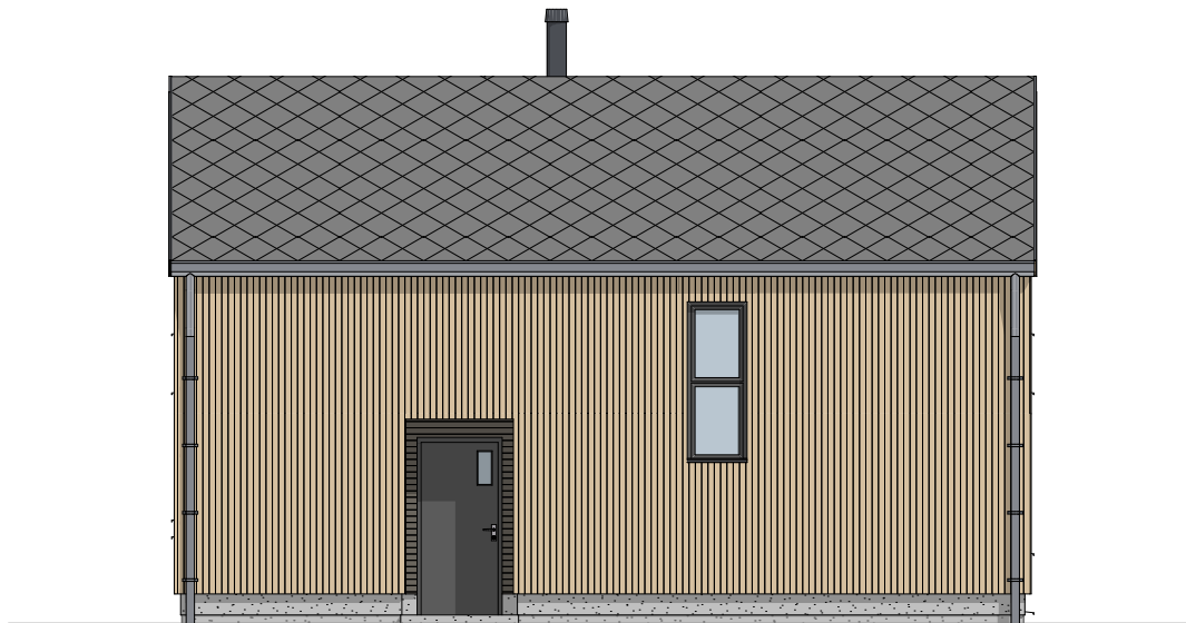
1:100 Fasade Nord Vest
