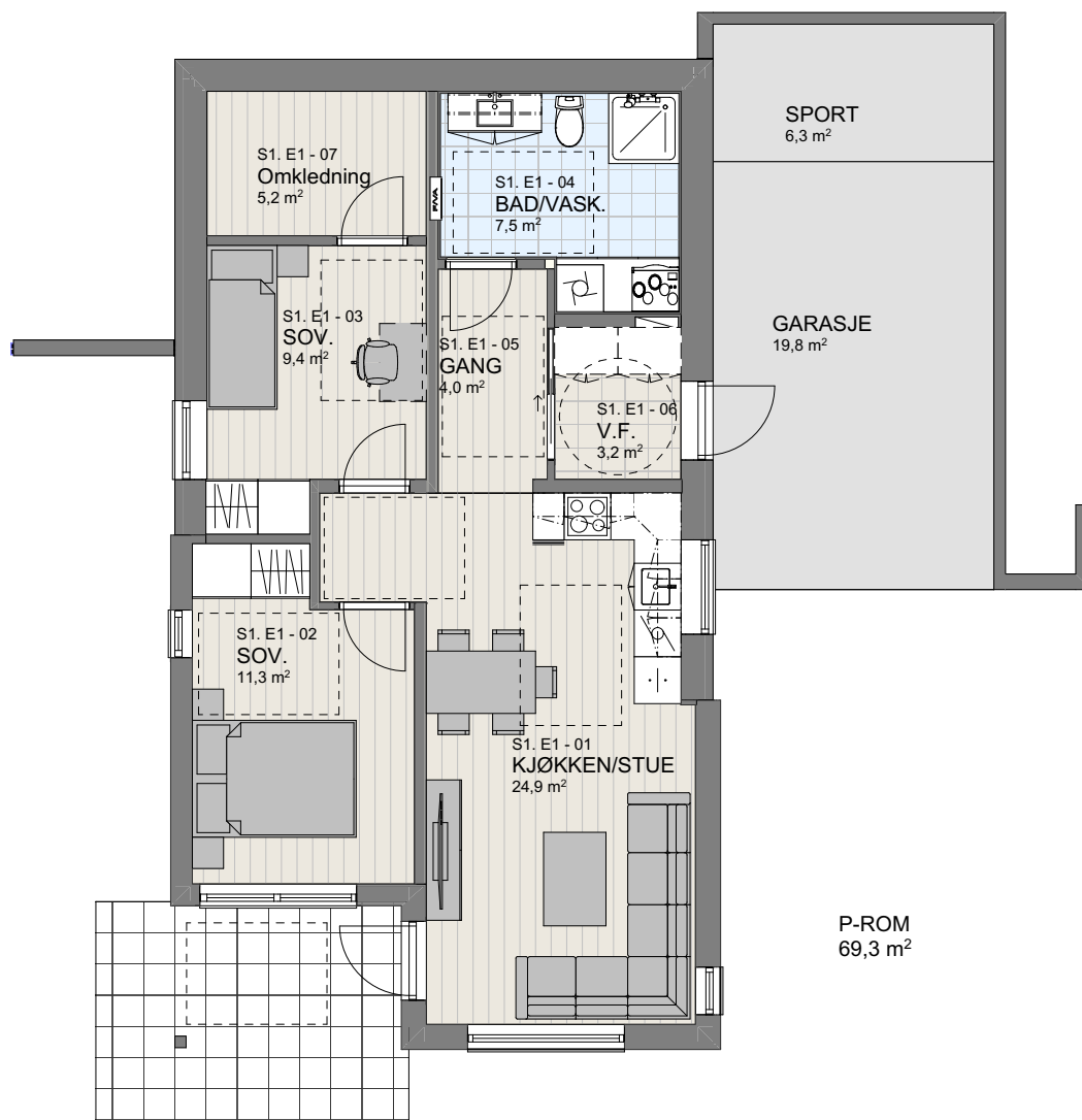
1:100 1. Etasje
