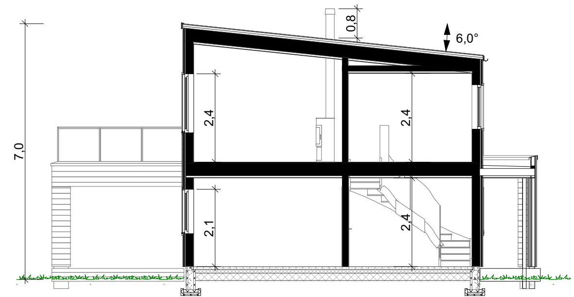
1:100 Schnitt B
