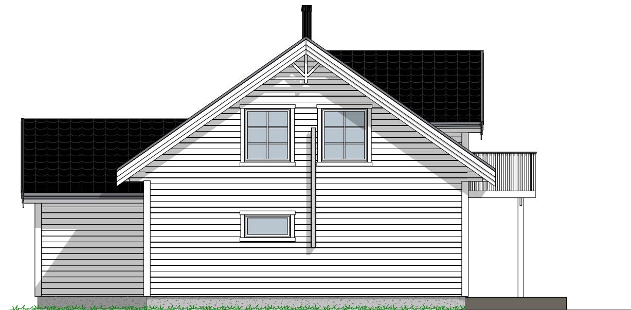
1:100 Fasade Øst
