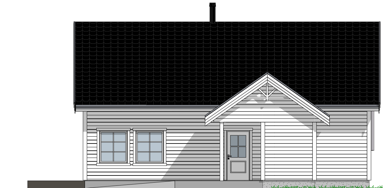
1:100 Fasade Sør
