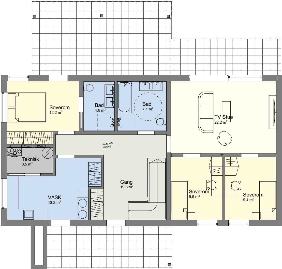
1:100 H. Etasje
