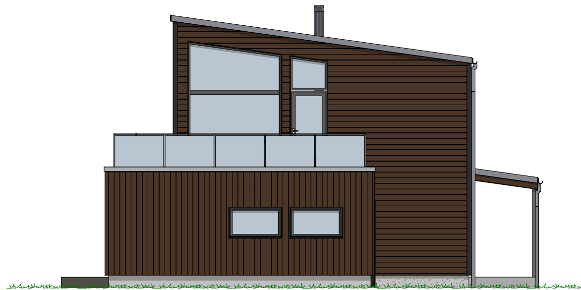
1:100 Fasade Sør
