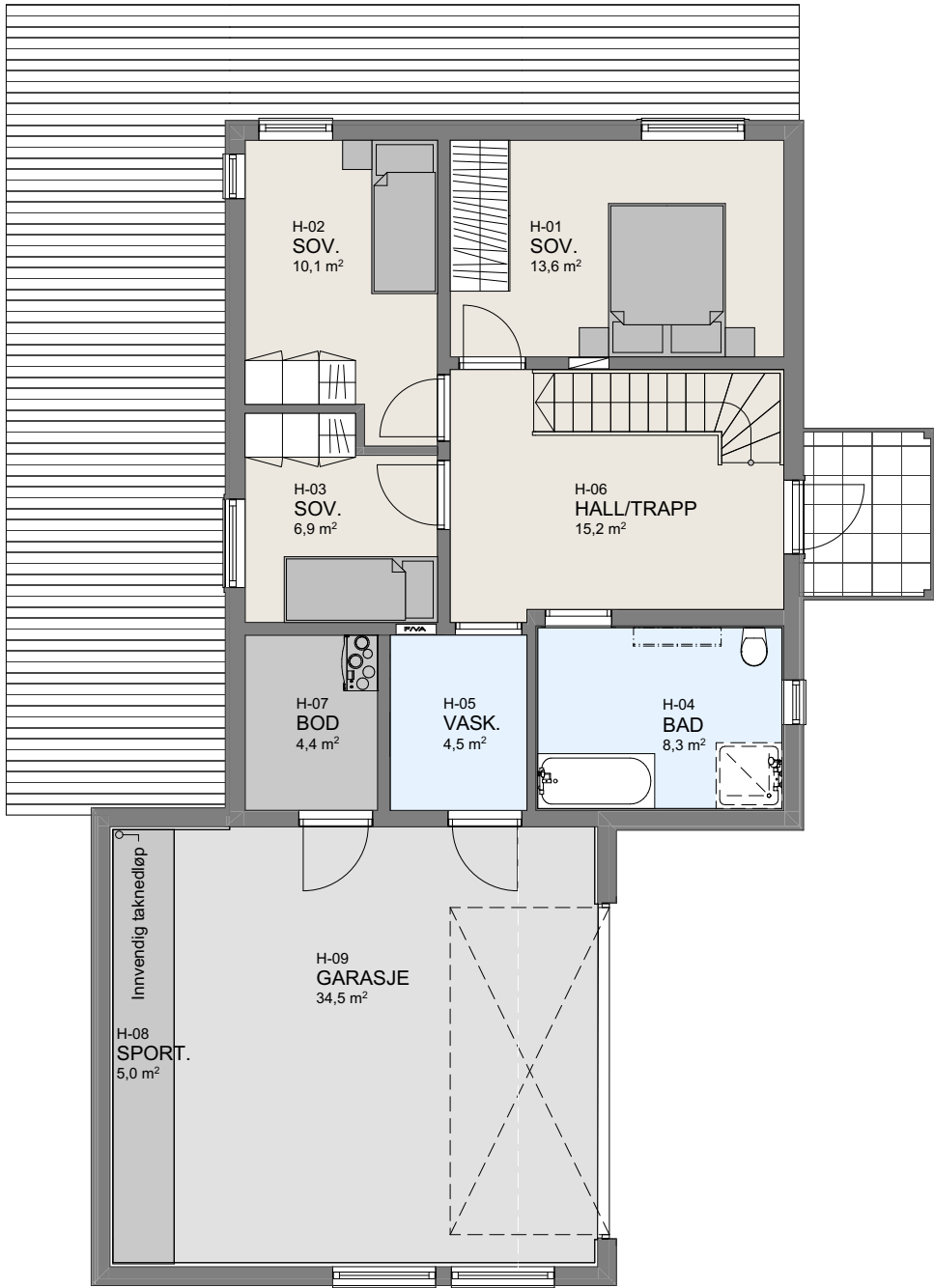
1:100 H. Etasje
