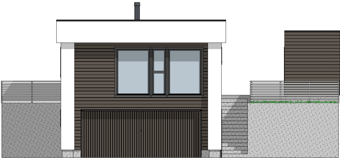
1:100 Fasade Sør
