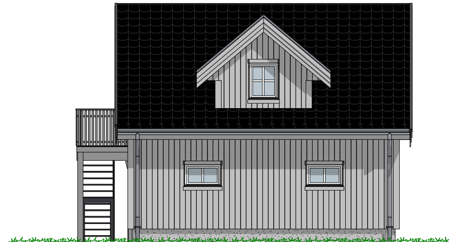
1:100 Fasade Nord Øst
