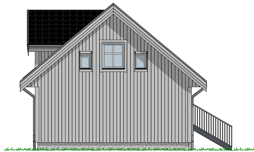
1:100 Fasade Nord Vest
