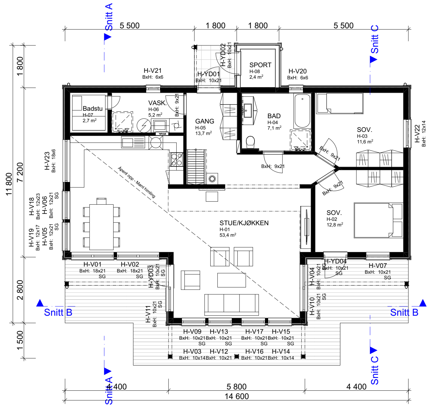
1:100 H. Etasje
