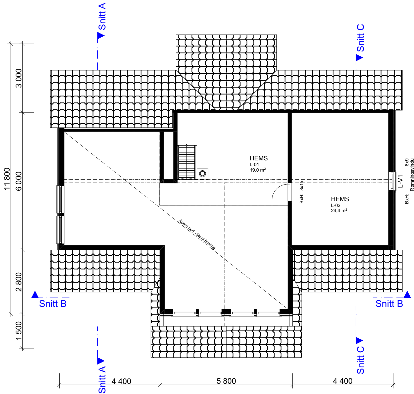
1:100 2.Etasje
