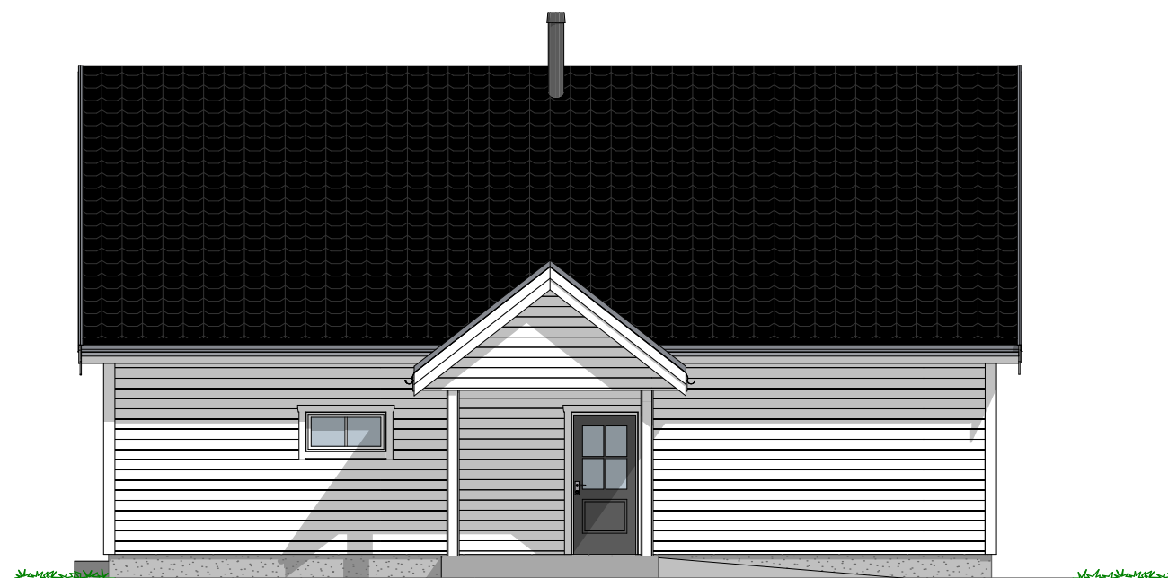
1:100 Fasade Øst
