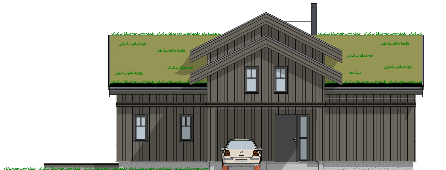
1:100 Fasade Sør
