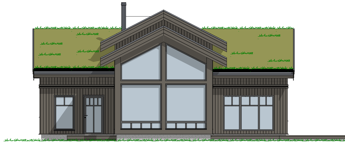
1:100 Fasade Nord
