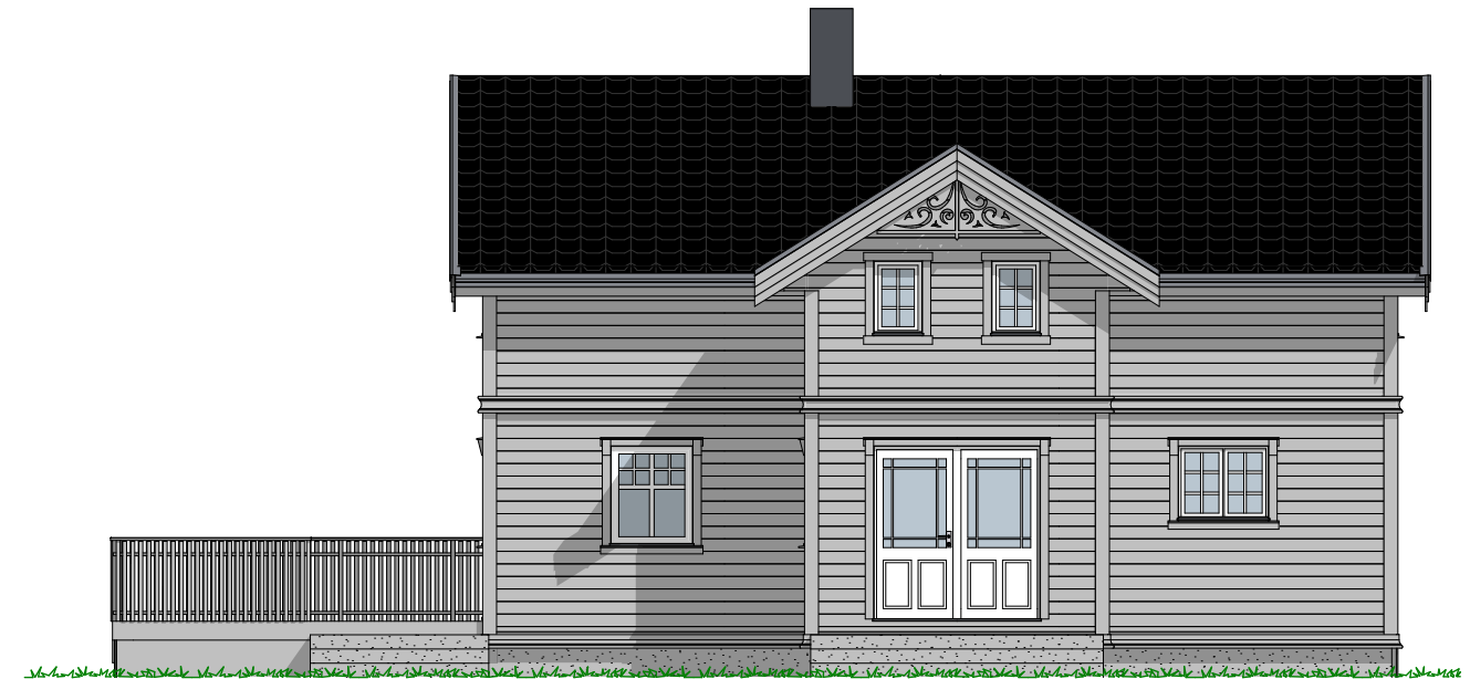
1:100 Fasade Sør Øst
