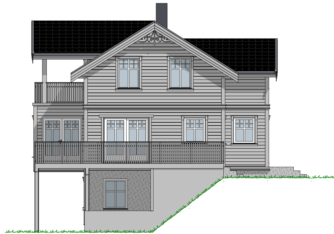
1:100 Fasade Sør Vest
