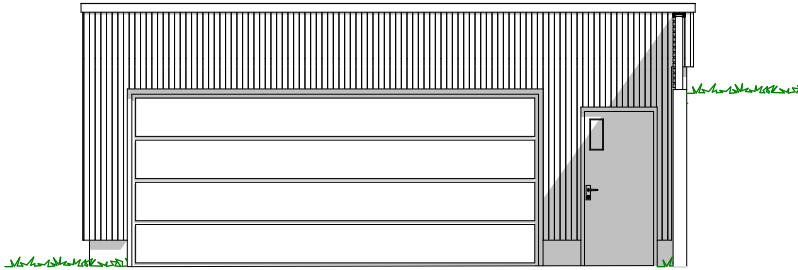
1:100 Fasade Sør
