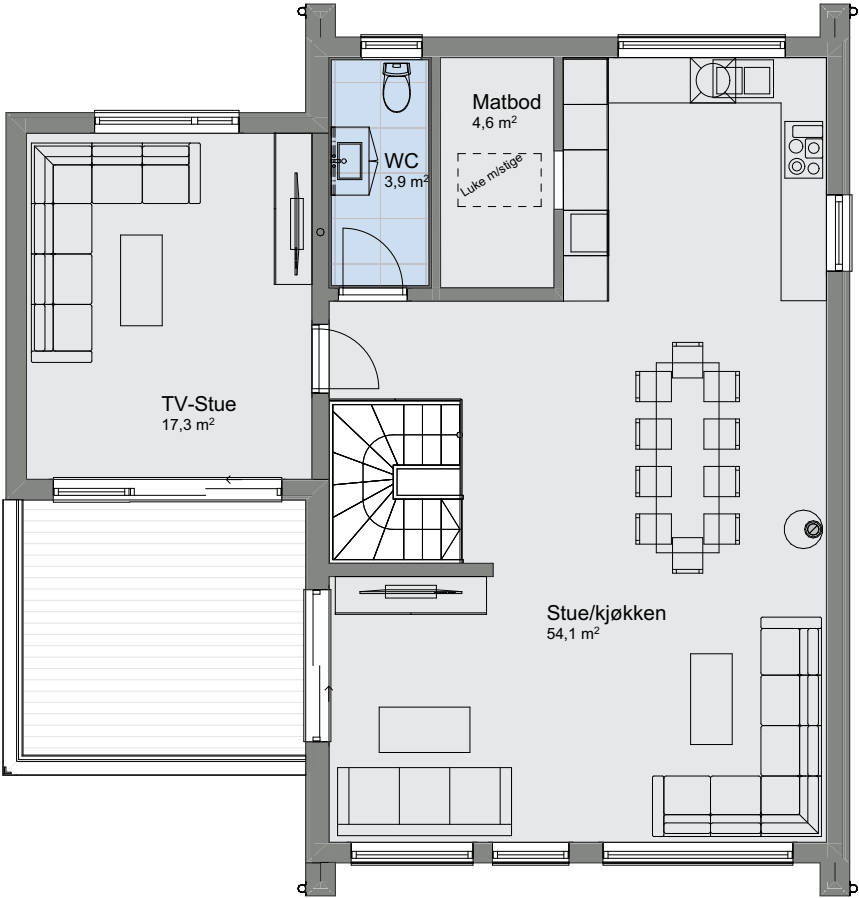
1:100 2. etasje
