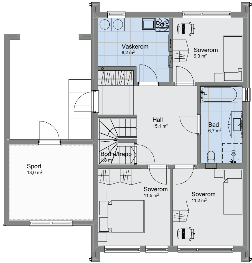
1:100 H. etasje
