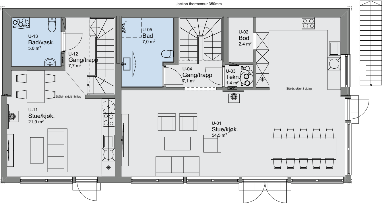
1:100 U. etasje
