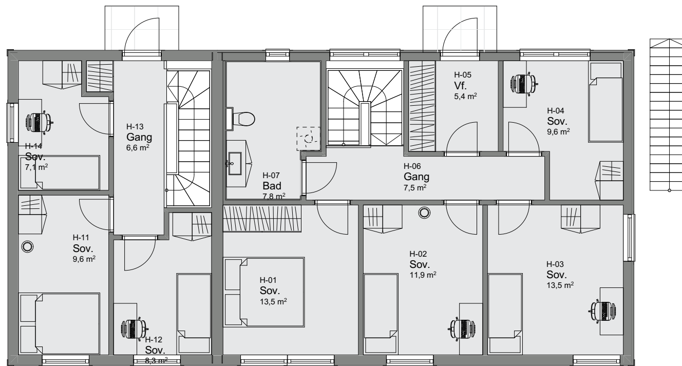
1:100 H. etasje
