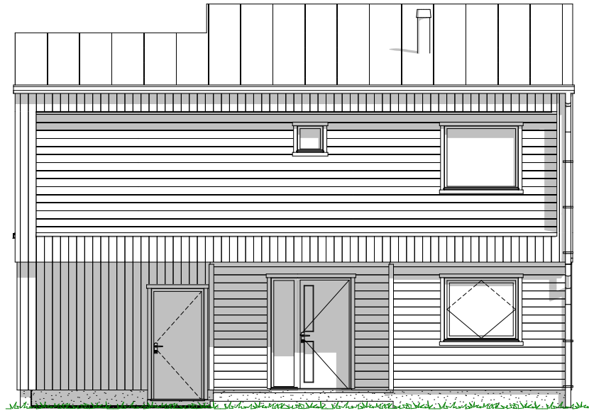
1:100 Fasade ØNØ
