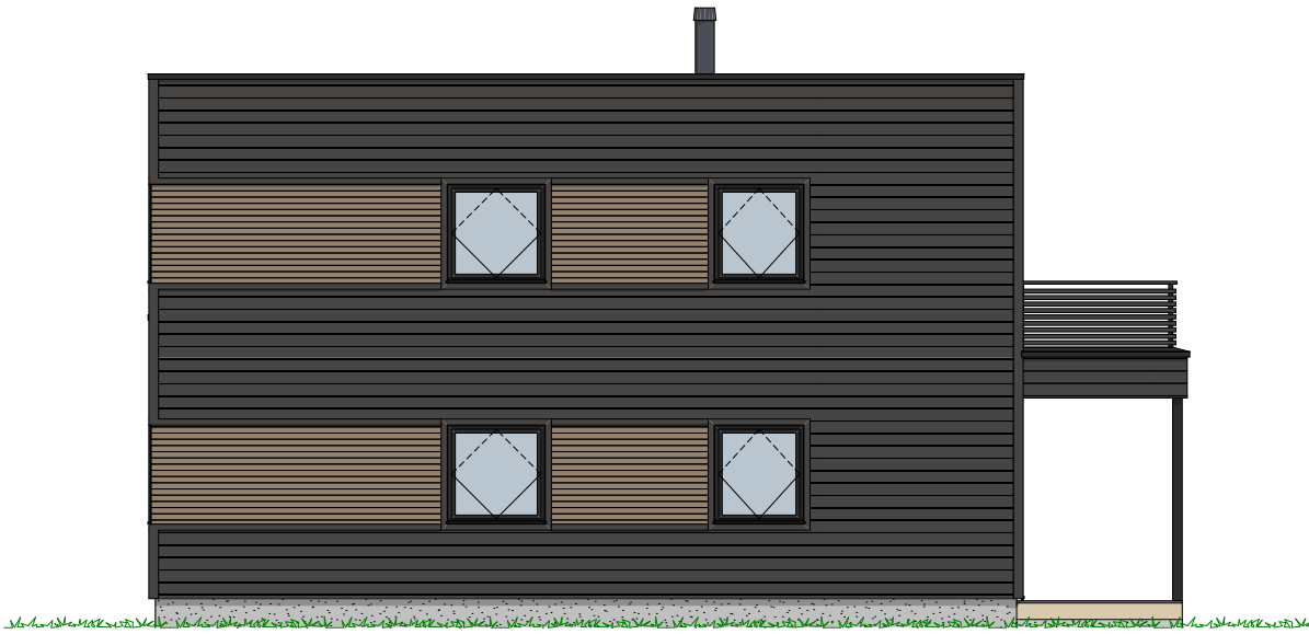
1:100 Fasade Nord
