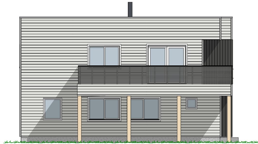
1:100 Fasade Vest
